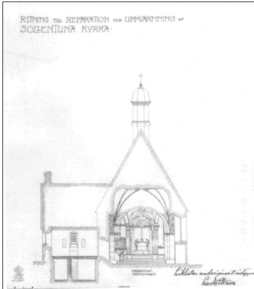
Sektion genom sakristian och koret, ark. Ludvig Pettersson 1902, ATA
