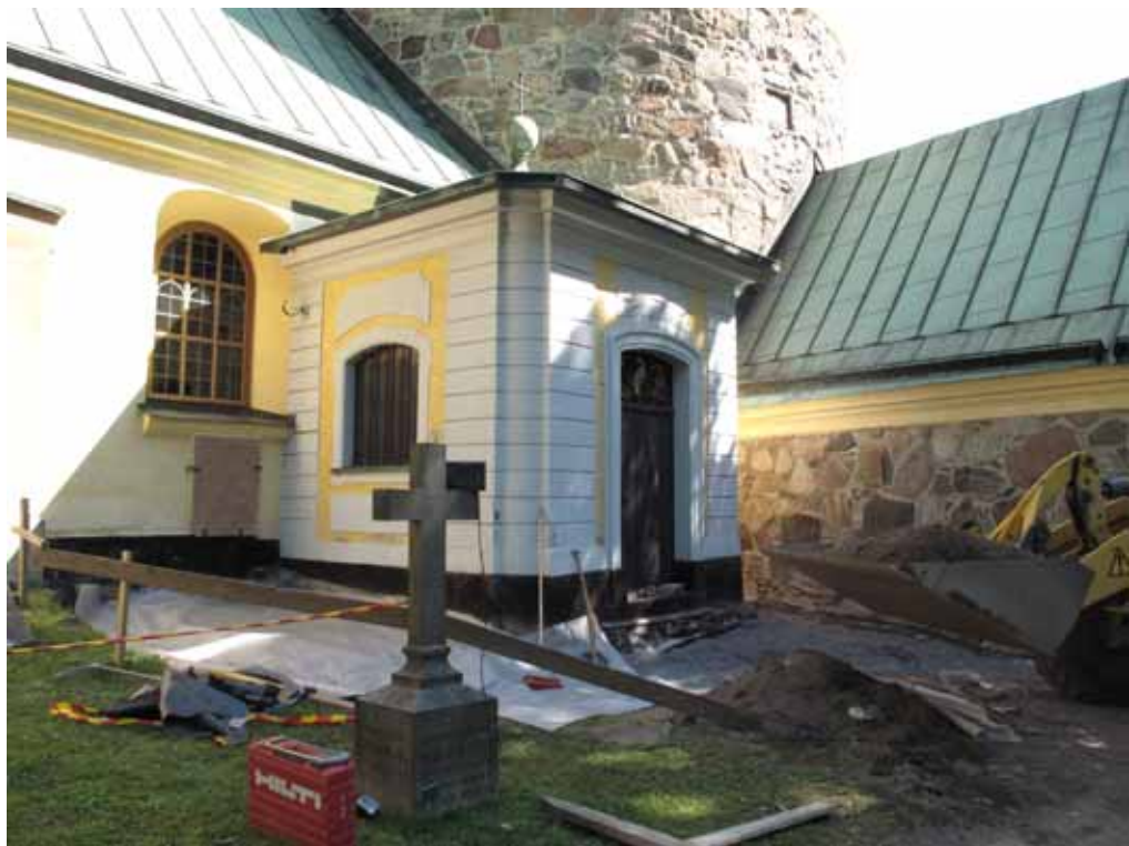
Dräneringsarbete pågår. Schakten är återfyllda. Foto Cecilia Pantzar Lp 20110529.
