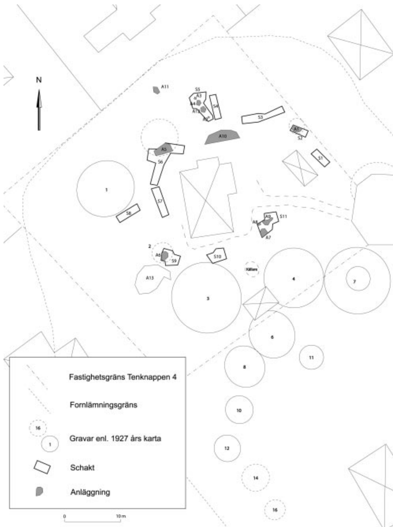
Fig 3. Schakt- och anläggningsplan, skala 1:250.
